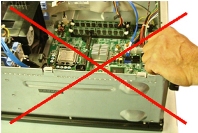
شکل ۹. اتصال زمین «فلز لخت» شاسی (غیرقابل قبول)
